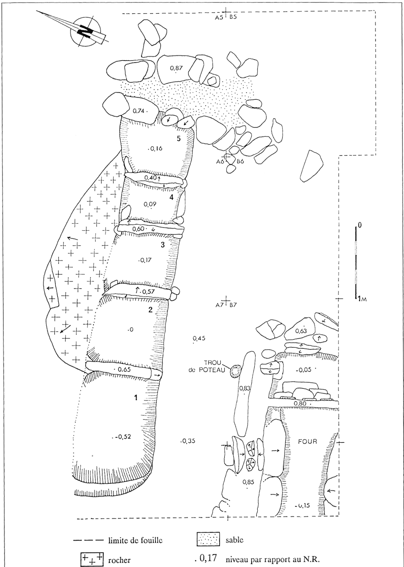
Fig. 2 : Landrellec en Pleumeur-Bodou (22) : plan général de la fouille et des structures de l'atelier de briquetages.
