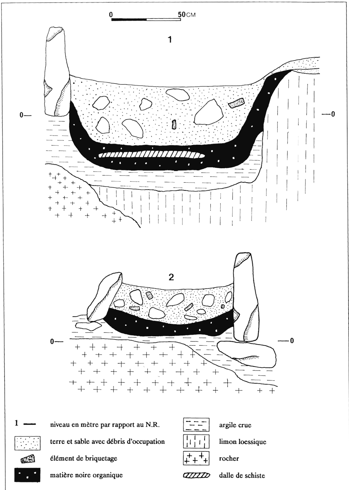
Fig. 8 : Landrellec en Pleumeur-Bodou (22) : coupes est/ouest des cuves n°1 et 2.
