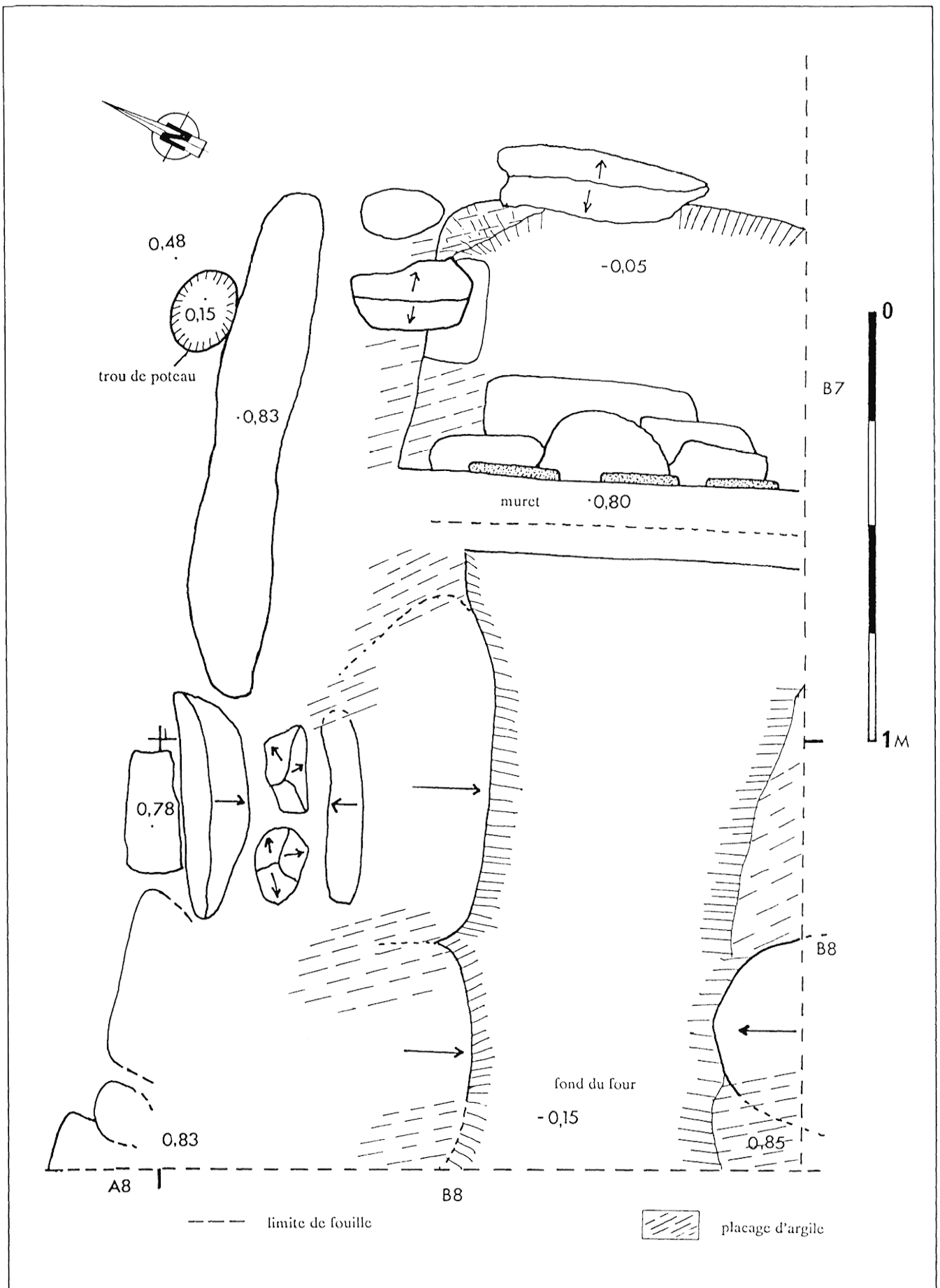
Fig. 5 : Landrellec en Pleumeur-Bodou (22) : plan détaillé du four.
