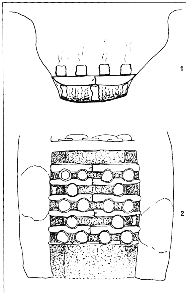
Fig. 9 : Landrellec en Pleumeur-Bodou (22) : hypothèse de reconstitution du chargement du four, 1 = en coupe, 2 = en plan.
