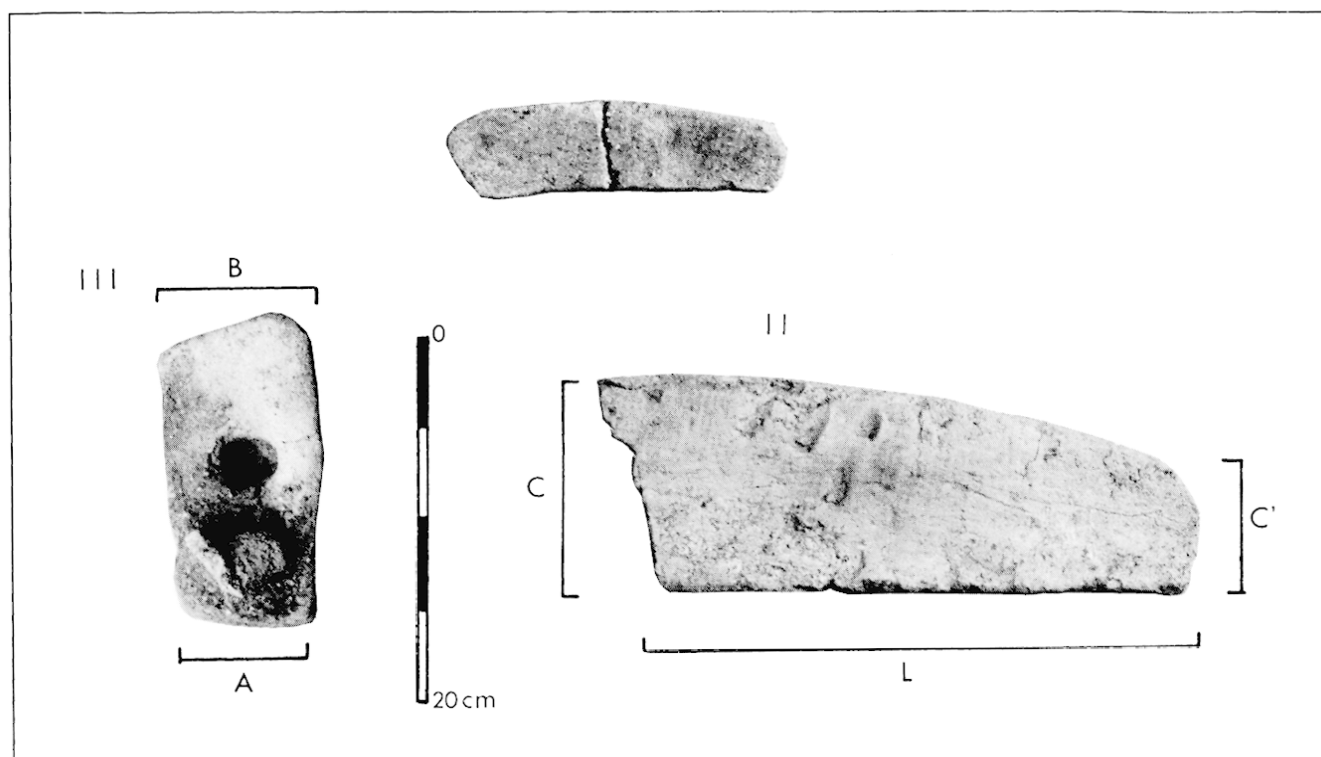
Fig. 10 : Landrellec en Pleumeur-Bodou (22) : briques provenant du four ; I : petit module, II : fragment de grand module, III : système d'attache avec tenon en argile.
