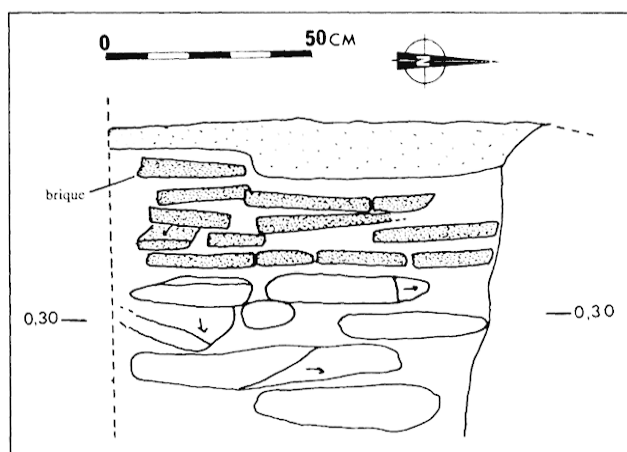
Fig. 7 : Landrellec en Pleumeur-Bodou (22) : élévation de la face est du muret de compartimentage du four.
